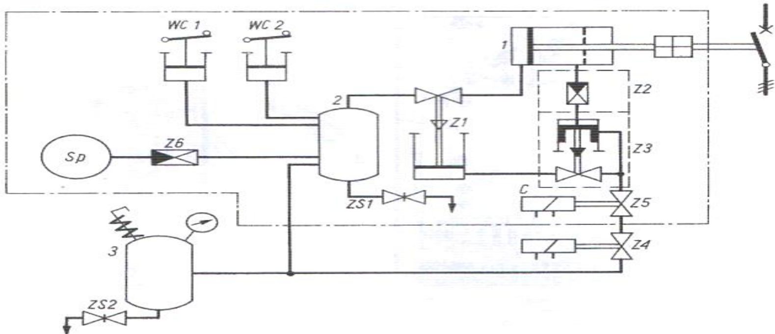
Rys. 19.9. Schemat układu pneumatycznego napędu pneumatycznego zasobnikowego NZP 1 — cylinder roboczy; 2 — zbiornik wyrównawczy; 3 — zbiornik dostawczy; Sp — sprężarka miniaturowa; Z1 — zawór główny; Z2, Z6 — zawory zwrotne; Z3 — zawór odcinający; Z4 — elektrozawór; Z5 — zawór blokujący; C — wyzwalacz zanikowy; ZS1, ZS2 — zawory spustowe; WC1, WC2 — wyłączniki ciśnieniowe
