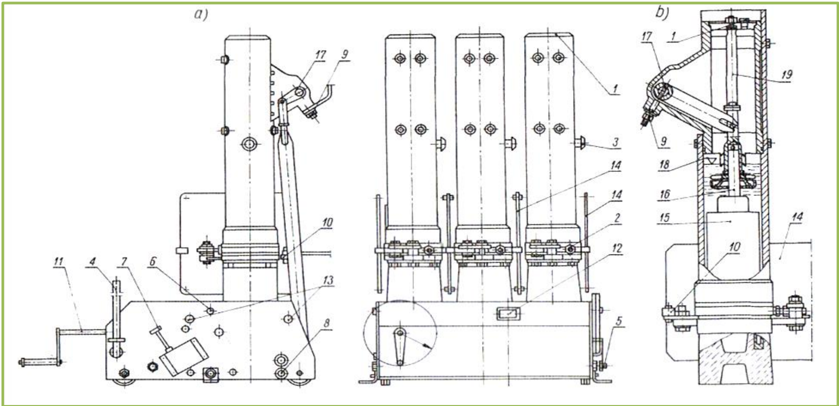
Rys. 19.5. Wyłącznik małoolejowy WMSWR10/6/3,5: a) widok wyłącznika; b) przekrój jednego bieguna
