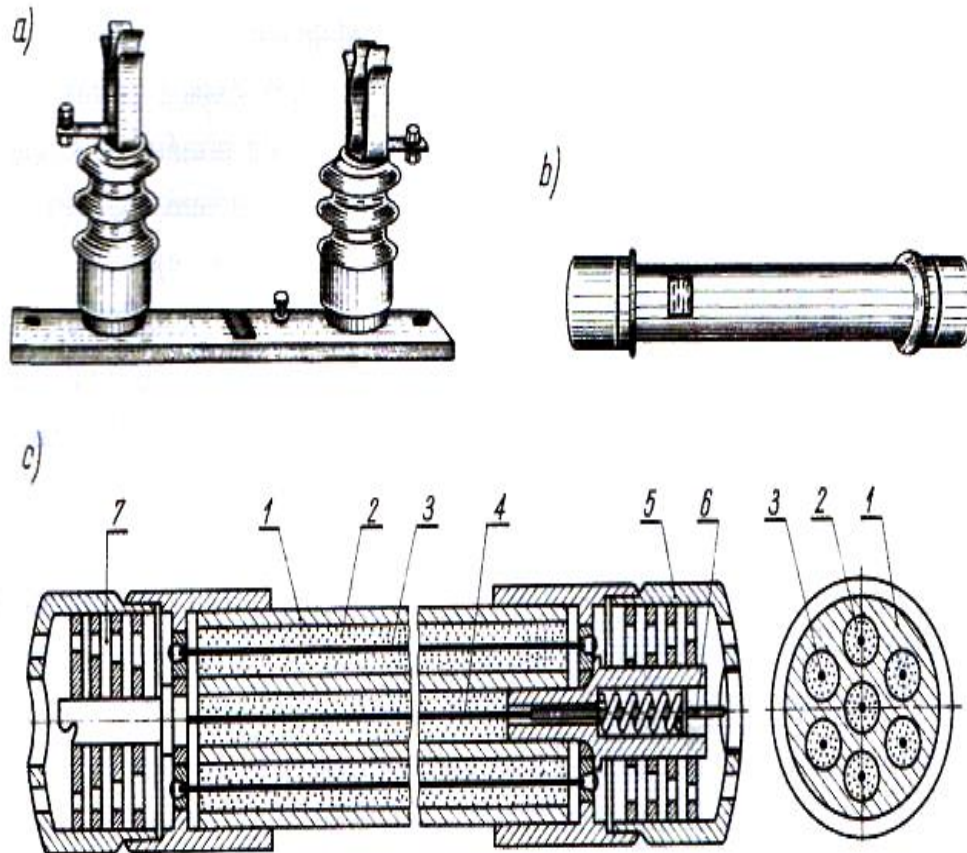
Rys. 19.12. Bezpiecznik wysokiego napięcia 8*15 kV o dużej mocy wyłączalnej:
